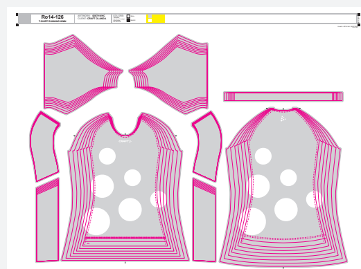
Productietekening van een Bike Jersey
